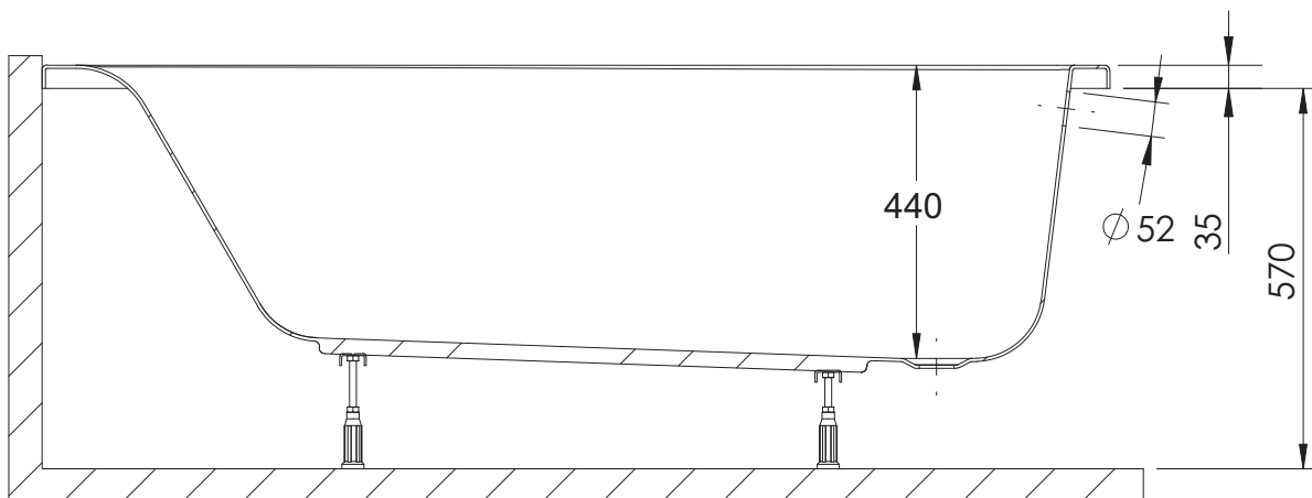
ŘEZ A-A
